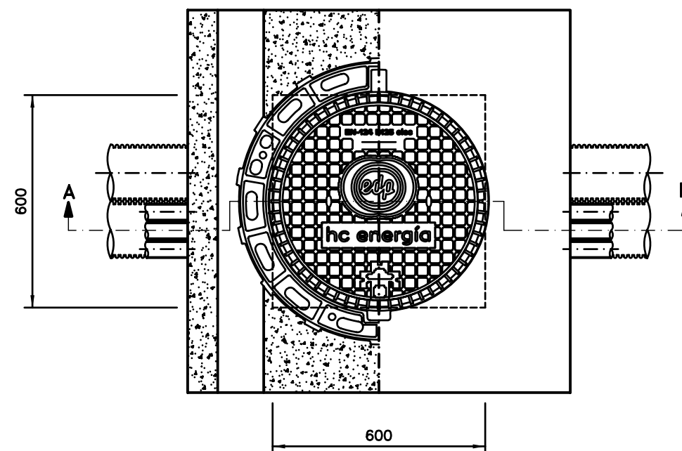
PLANTA
