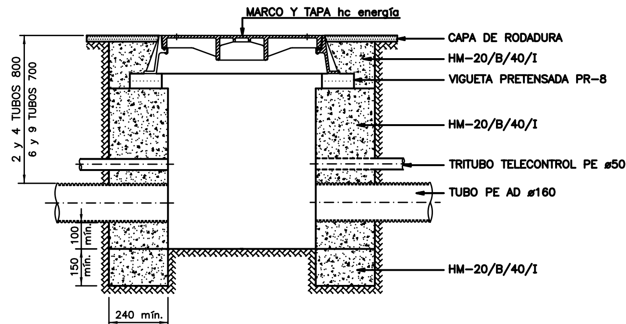
SECCION A-B
